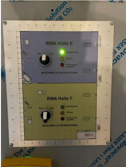
Bedienungstableau Air Kraft
