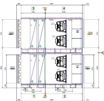
5 Stück Rückkühler mit je 42'000 m3/h
