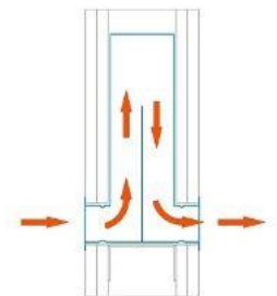
Gehäuse mit schmalem Schlitz
